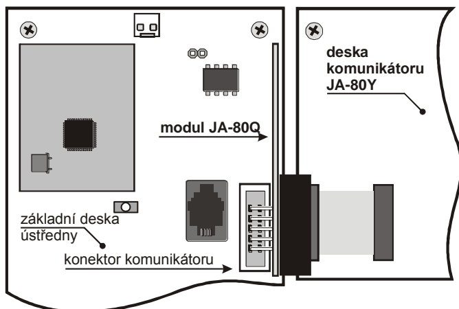
Obr. 1 Zapojení modulu
