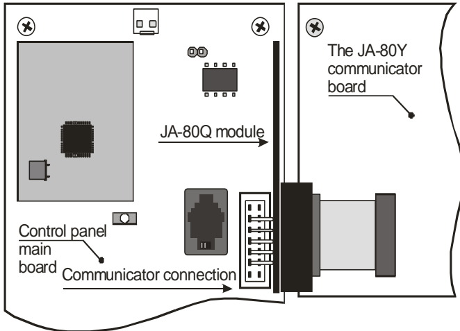
Fig. 1 Module wiring
