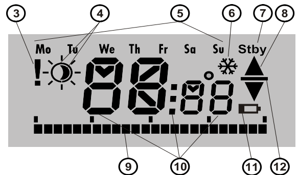
Afbeelding 3: 3 – Interne instellingen van de invoer vanuit een fout van de SW/communicatie van de F-Link; 4 – Symbolen voor de comfort en economische temperatuur;
